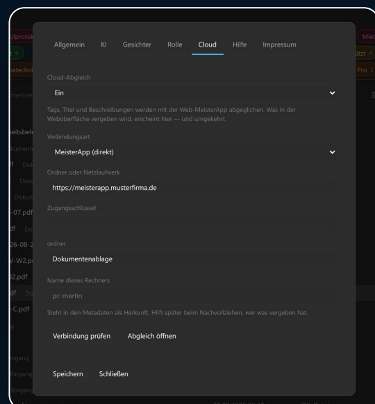
Der Cloud-Reiter: Verbindungsart und Zugangsdaten – neben MeisterApp (direkt) auch SFTP, FTPS, FTP, WebDAV, S3 und Netzlaufwerke.
